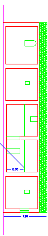
SEZIONE 'XXX'
